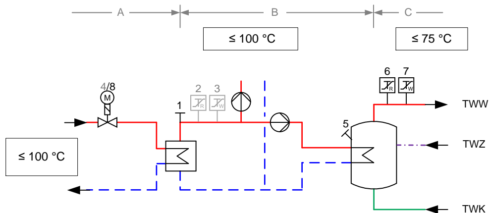
Abbildung 13: zur Tabelle 6: Erforderliche sicherheitstechnische Ausrüstung nach Zeile 2; grau dargestellte Komponenten nicht erforderlich
