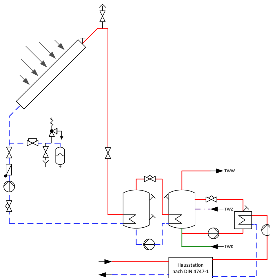
Abbildung 17: Solaranlage mit Pufferspeicher und Trinkwassererwärmer mit außen liegendem Wärmeübertrager für die Nachheizung
